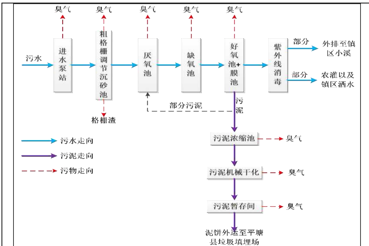
图2-1 运营期污水处理工艺流程及产污环节图
