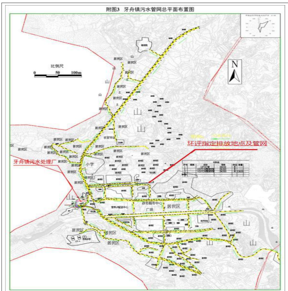
环评要求排放指定位置及管网图
