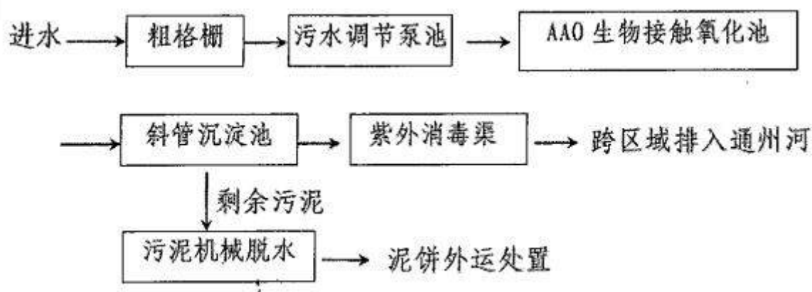
图2-1 污水处理工艺流程及产污环节图
