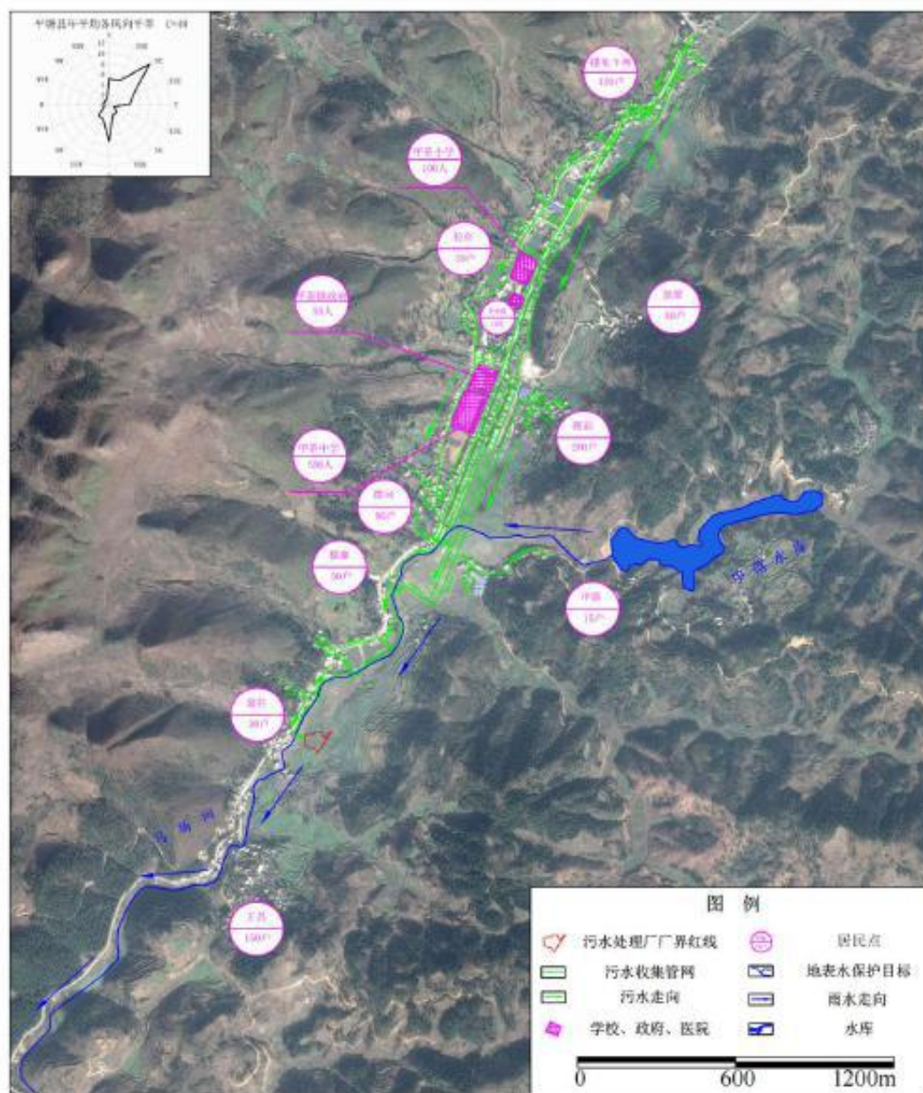
附图3 污水管网总平面布置图
