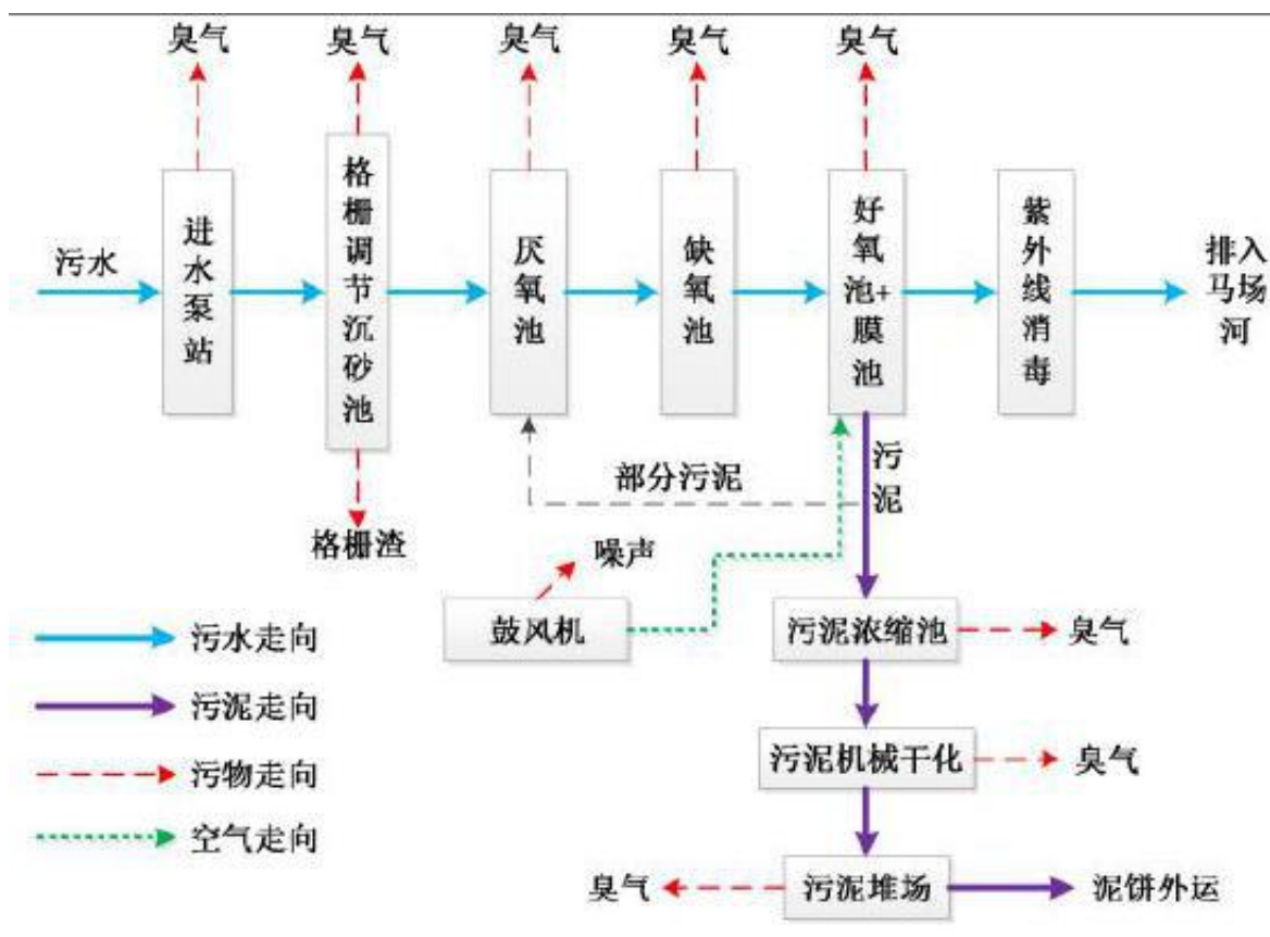
图 1-1 营运期污水处理工艺流程及产污环节图
