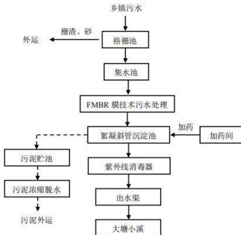
图2-2 污水处理工艺流程及产污环节图
