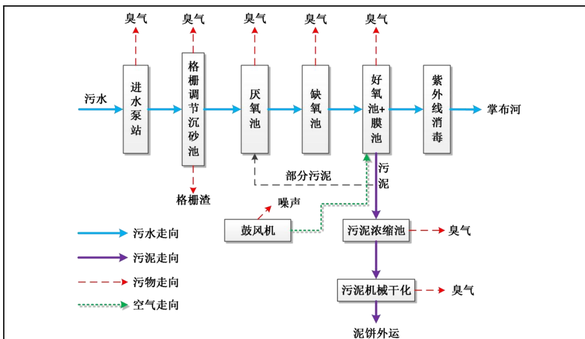
图 2-1 运营期污水处理工艺流程及产污环节图
